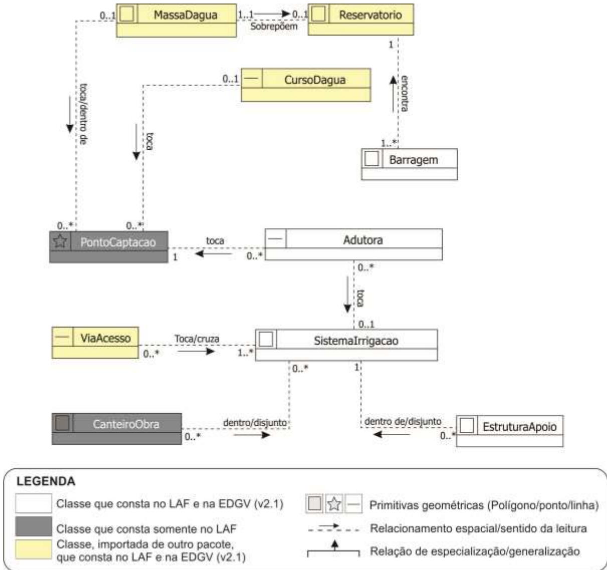
Figura 1- Modelo de dados referente à tipologia Irrigação.
