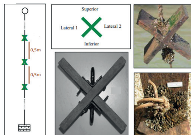
Figura 24. Substrato artificial de madeira em forma de "X" para amostragem de indivíduos recrutas e adultos do mexilhão-dourado. Fonte: Pereira et al. (2012b), com autorização dos autores e editores.
