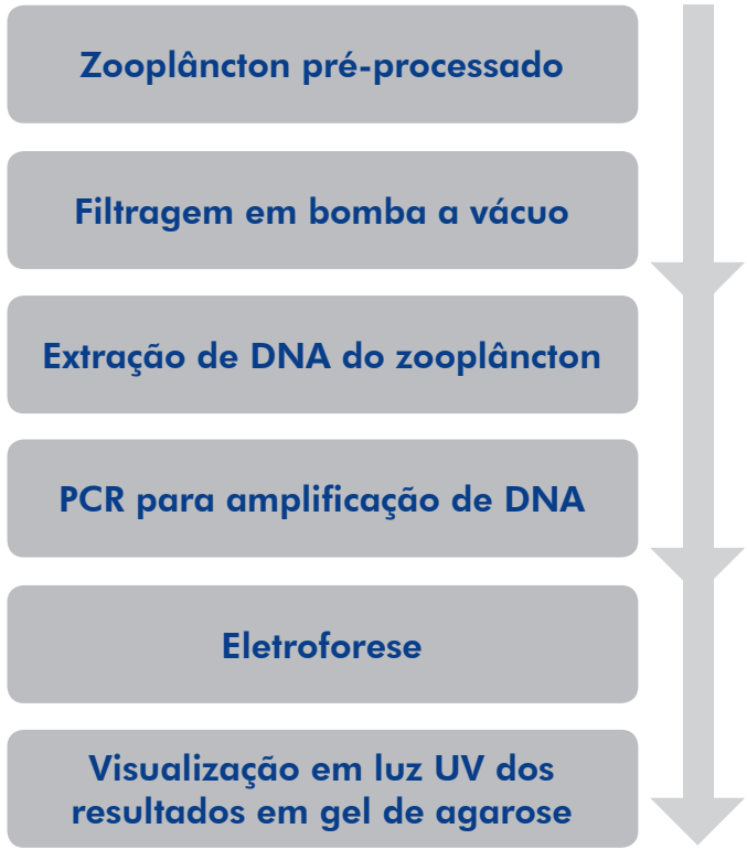
Figura 19. Etapas do protocolo PCR de detecção de presença e ausência de larvas do mexilhão-dourado. Fonte: Tschá et al. (2012).
